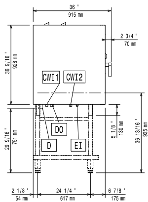
Zij aanzicht
